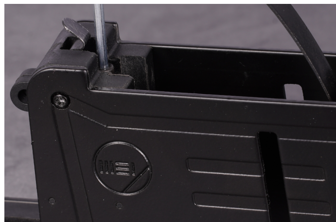
Feinjustierung der Verschlussfeder
